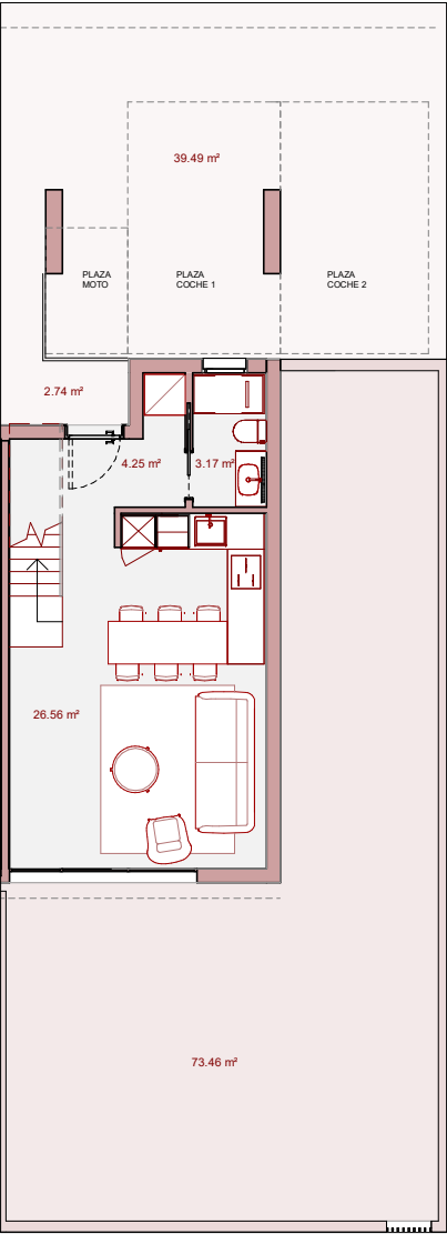
Planta Baja
