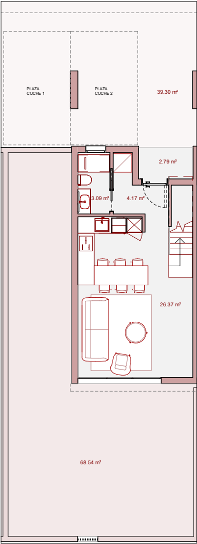
Planta Baja
